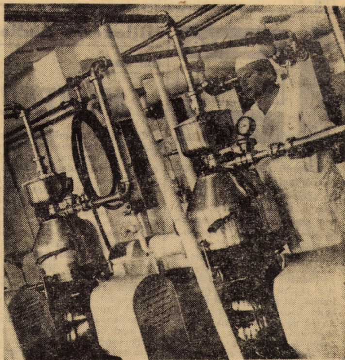
Întreprinderea de industrializare a laptelui Sibiu. După recepția din bazine, înainte de-a ajunge la pasteurizare, laptele este trecut prin instalații speciale de curățare a impurităților
