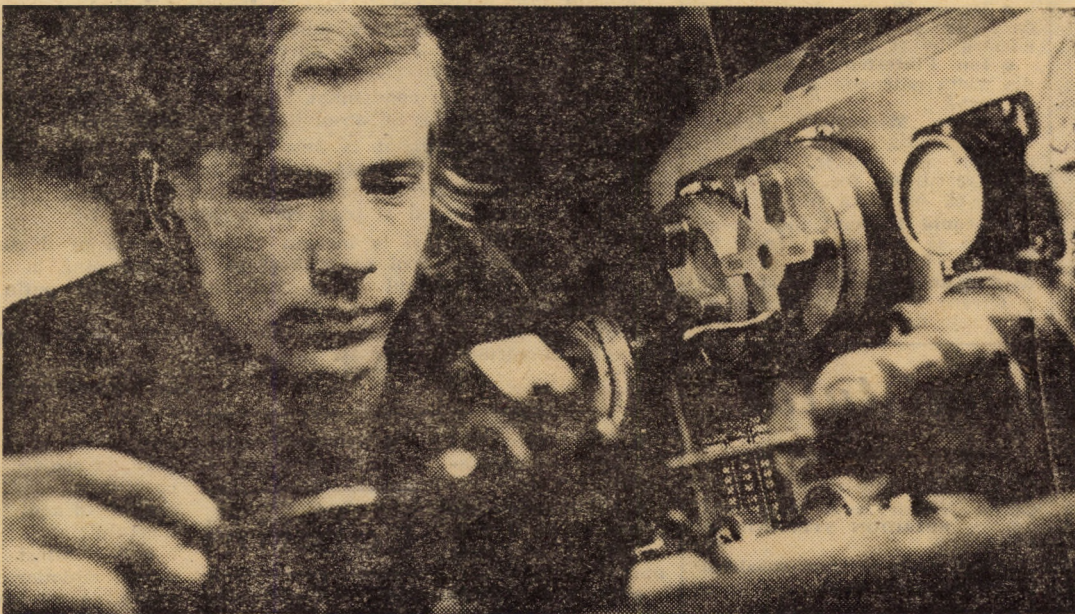
În atelierul sculărie al întreprinderii de șuruburi Mediaș, utecistul Martin Gross, rectificator cu o bună pregătire profesională, execută — la un utilaj de înaltă precizie — lucrări de suprafinisare la matrițe din metal dur, necesare presării la rece a șuruburilor
