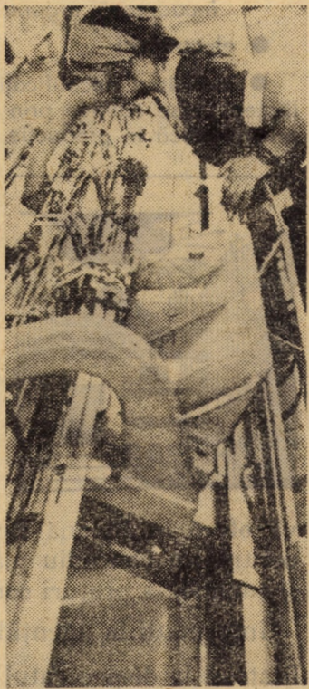
Mașină rectilinie automată de tricotat, cu o productivitate de 100 perechi mînuși în 8 ore — utilaje din cele mai perfecționate în obținerea de modele Jaquard în culori la întreprinderea de mînuși și ciorapi Agnita
