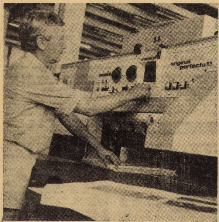
Un nou utilaj de înalt randament în secția legătorie a Întreprinderii poligrafice Sibiu: mașina de tăiat cu comandă program deservită de comunistul Nicolae Bratu. Foto: FRED NUSS
