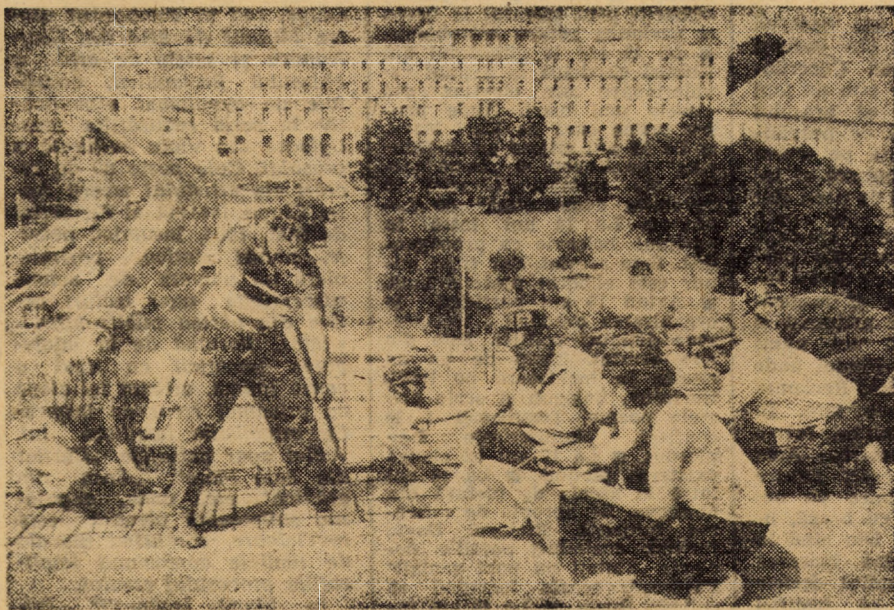
Secvență de lucru surprinsă pe șantierul nr. 3 lotul II Sibiu: magazinul universal (str. Gheorghe Gheorghiu-Dej). Echipa de dulgheri, condusă de Ion Schenn lucrează la montarea cofrajelor și a prefabricatelor la ultimul nivel (terasă). Cum reiese din angajamentul echipei, pînă la sfîrșitul acestui an vor fi terminate toate lucrările de dulgherie
