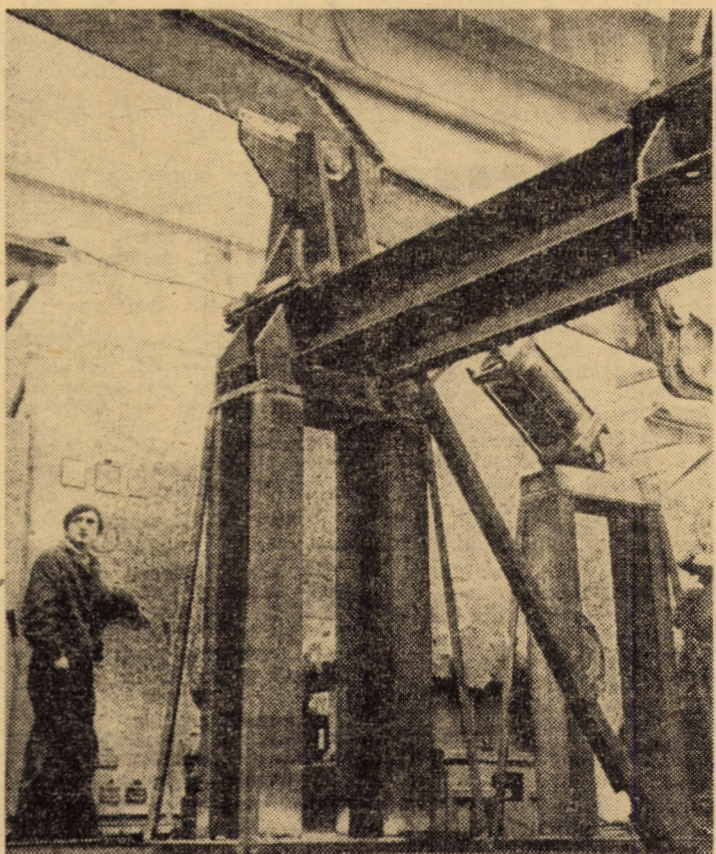
Secția II mecanică, atelierul montaj al întreprinderii „Independența” din Sibiu. Destruitorul de țigle destinat industriei siderurgice („Oțel inox” Tirgoviște) aflat pe bancul de probă Foto: FRED NUSS
