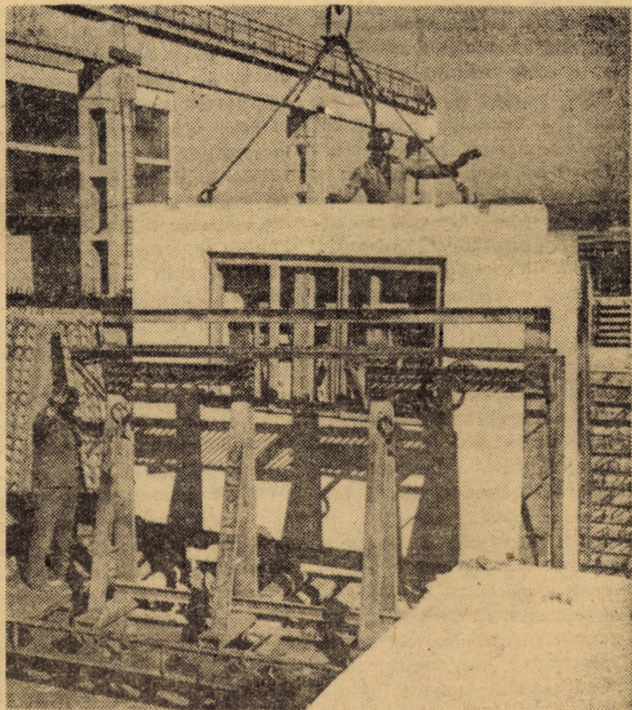
La noua bază de producție a I.C.M.J. Sibiu se execută mecanizat panouri prefabricate destinate construcțiilor de locuințe.
