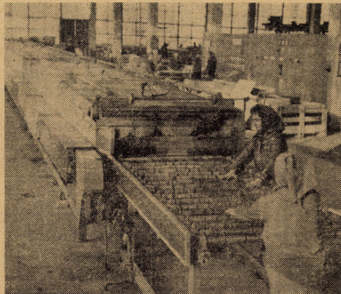
Fabrica de geamuri Mediaș. Linia continuă de geam securizat plan
