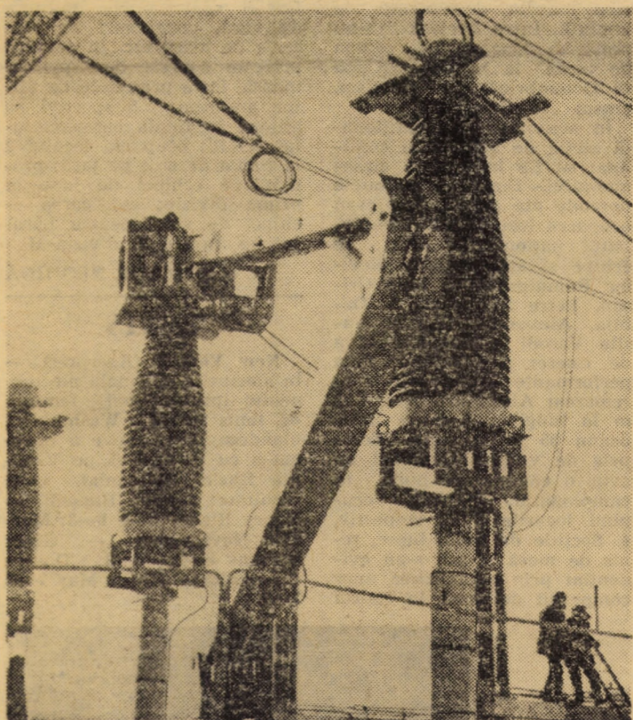
Revizia unui întrerupător de 400 KV a stației Sibiu-Sud Foto: FR. NUSS
