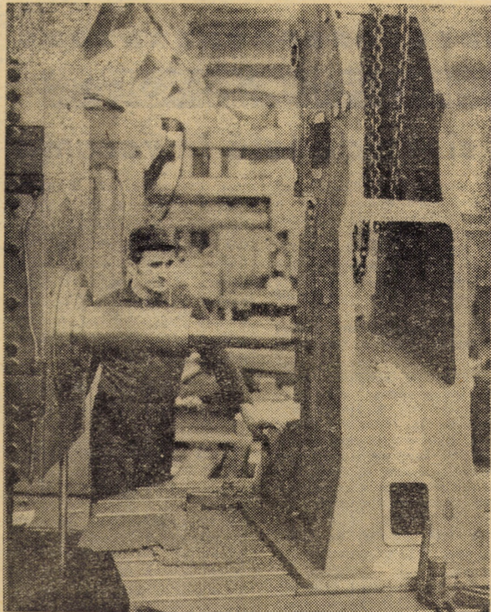
Întreprinderea „Mecanica” Sibiu. Comunistul Ilie Minzat la locul său de muncă din secția prelucrări prin așchiere deservind o o mașină de frezat, alezat, strunjit și găurit
