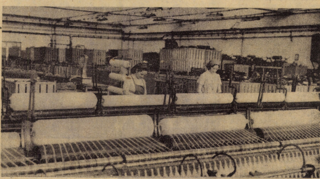
Vedere de ansamblu a secției filatură a fabricii „Progresul” din Orlat. În fotografie: grupul de selfactoare la care se produc fire pentru stoffe de mobilă în 7 culori diferite Foto: FR. NUSS
