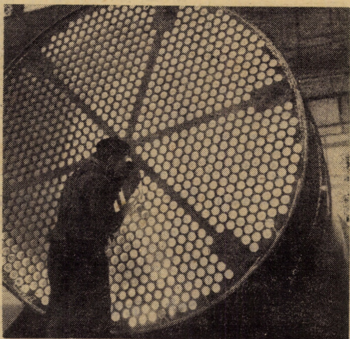
Unul din utilajele „gigant” produs de cazangeria grea a întreprinderii „Independența” Sibiu — evaporator de Ø 2 500 mm destinat Combinatului de aluminiu Tulcea
