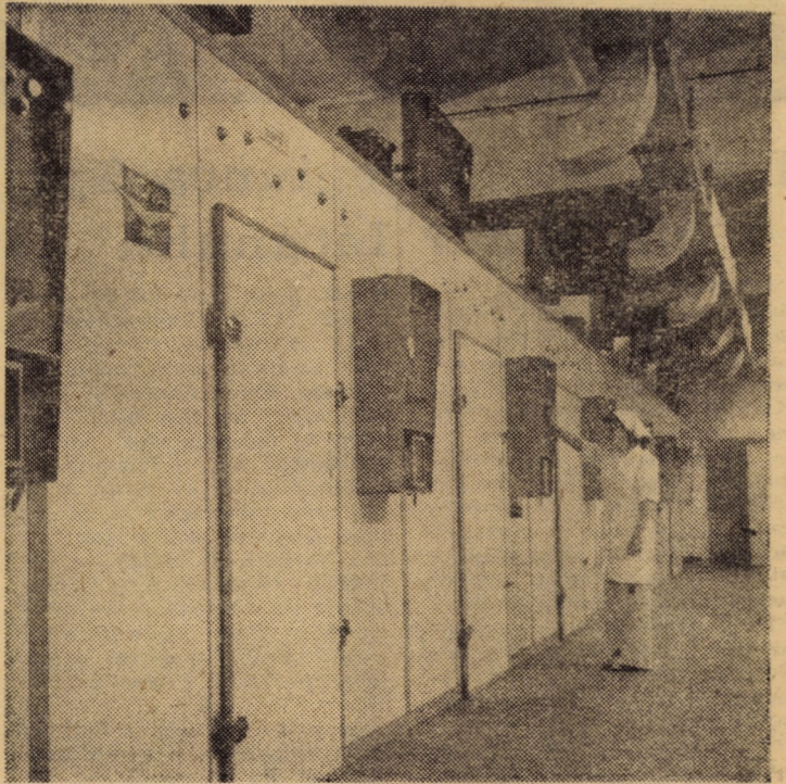
La centrul de incubatie al întreprinderii „Avicola” de stat Sibiu, temperatura, umiditatea și ventilația sînt dirijate automat. Operatori de înaltă calificare profesională supraveghează aparatul de control și intervin ori de cîte ori apar situații deosebite.
