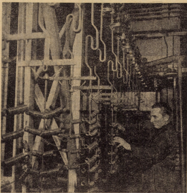
La I.P.A. Sibiu, preocupările pentru realizarea unor utilaje prin efort propriu se confundă deopotrivă cu cele pentru materializarea ideii de nouă calitate. Dovadă, baia de vopsire prin electroforeză, prezentă în imaginea noastră
