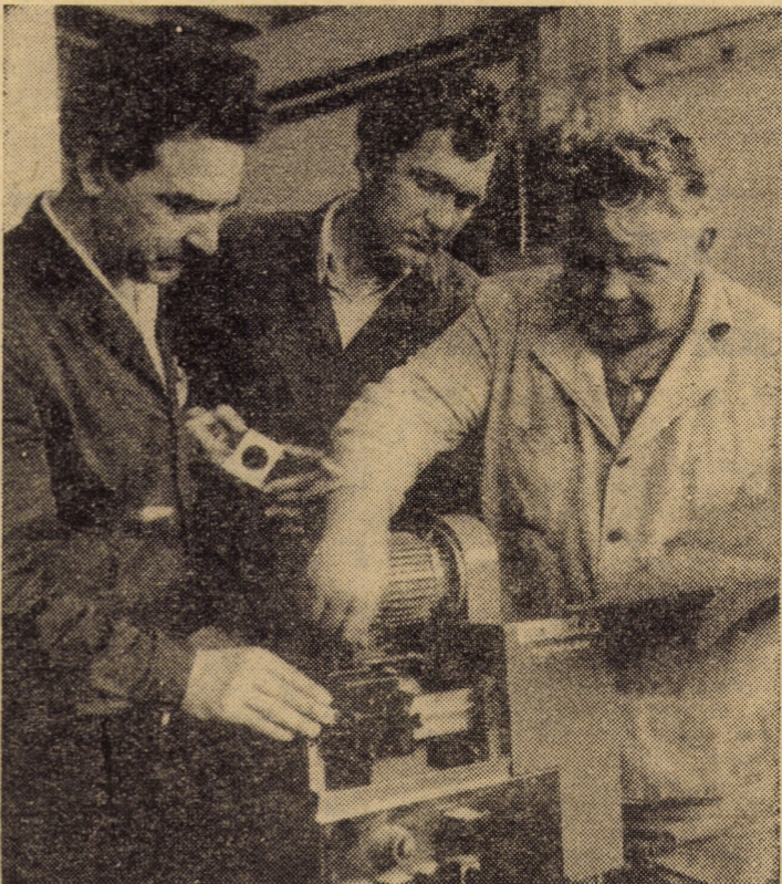
În atelierul de autoutilare al întreprinderii „Flamura roșie” Sibiu, unitatea a II-a monobloc a fost realizată o mașină semiautomată de ascuțit ace cu virf special pentru industria pielăriei, prin care se va elimina în bună parte importul la aceste produse. În fotografie: maistrul Iosif Tintea, lăcătușii Günther Acudi și Gavril Șildan asistind la probele tehnologice
