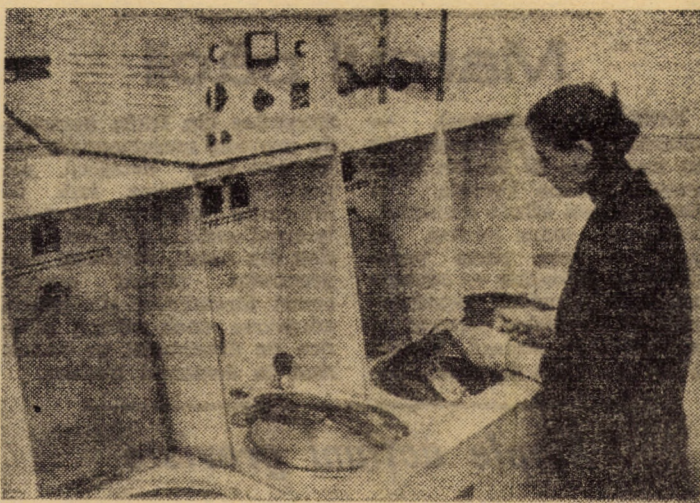
Reproducem în instantaneul nostru fotografic, unul dintre utilajele de mare productivitate, aflate în dotarea întreprinderii sibiene „Flamura roșie”: instalația de degresare prin acțiunea ultrasunetelor a virurilor metalice pentru rezervele de pastă
