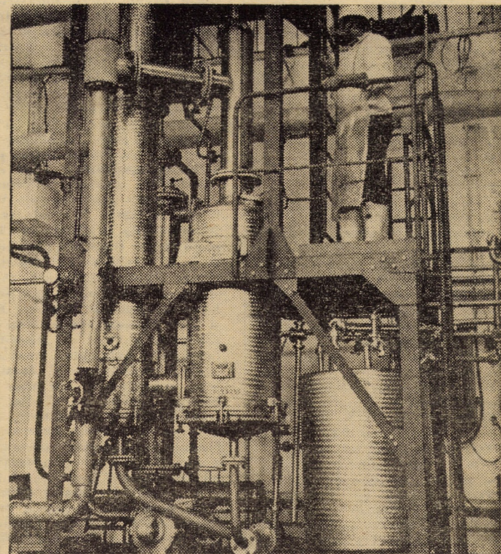
Noua instalație pentru concentrarea laptelui, dată recent în funcțiune în atelierul de produse proaspete al Întreprinderii de industrializare a laptelui Sibiu Foto: FRED NUSS
