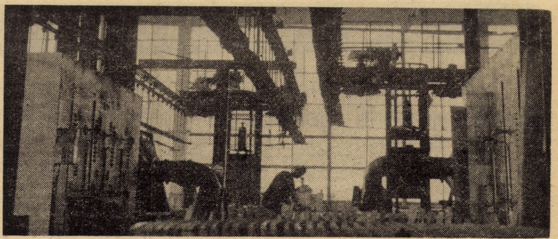
Linia transportoare la instalația de curbare din atelierul geam securit al Fabricii de geamuri Medias Foto: FRED NUSS
