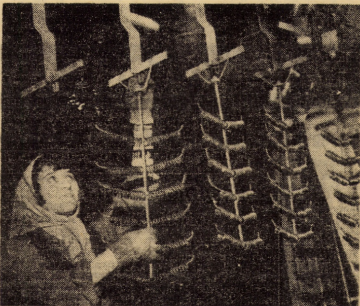
Linia de vopsit prin electroliză - una din instalațiile moderne realizate prin autodotare la întreprinderea de piese auto Sibiu
