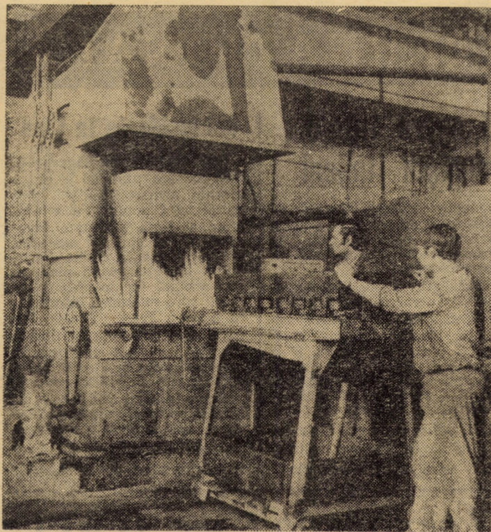
În atelierul tratamente termice al I.M.A.I.A. Sibiu, de cca. două luni a fost dată în funcțiune o nouă și modernă linie de tratamente termice cu atmosferă controlată. Prin folosirea noilor utilaje, calitatea semifabricatelor s-a îmbunătățit simțitor. Foto: FRED NUSS
