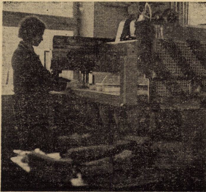
La mijlocul lunii ianuarie a.c., în cadrul unității a II-a de la F.I.P.A. — secția încălțăminte — a fost pusă în funcțiune o mașină de croit în mai multe straturi — utilaj modern care înlocuiește munca a 8 muncitori Foto: FRED NUSS
