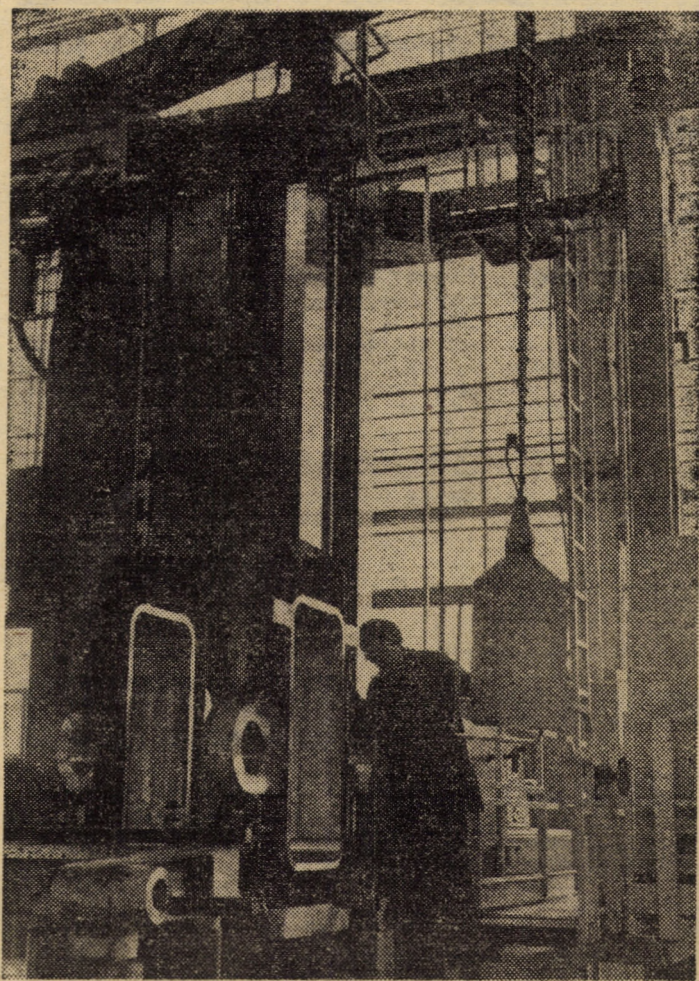
Printre utilajele de mare capacitate și tehnicitate de la „Independența II” se numără și acest borwerk, utilaj cu programare numerică, deservit de strungarul Ion Munteanu. Foto: H. BUCHFELNER
