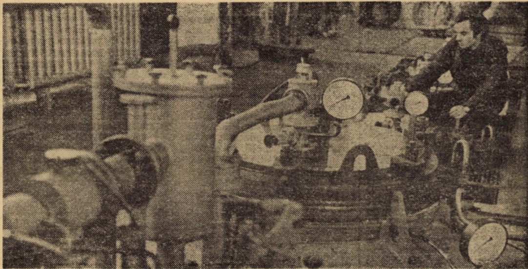
Instalații complexe, de înaltă tehnicitate pentru reacoacerea în vid a sirmei, din secția metal II a întreprinderii „Flamura roșie” Sibiu
