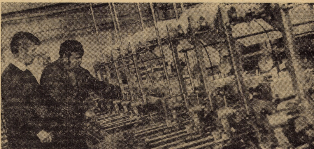
O realizare de ultimă oră a colectivului de muncitori, tehnicieni și ingineri de la întreprinderea „Balanta” II, Sibiu: mașina de canetat fire groase — utilaj cu performanțe mult îmbunătățite față de cele importate, la montajul căreia și-a adus o importantă contribuție echipa condusă de Ioan Szalmari.
