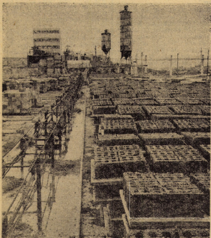
Secția de prefabricate blocuri mici din beton cu agregate ușoare a întreprinderii „Record” Sibiu. Această secție valorifică (sezonier) în mod superior spărturile de cărămidă Foto: FRED NUSS
