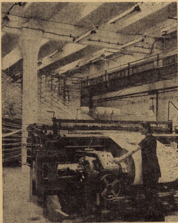
Unul din utilajele recent date în funcțiune la întreprinderea „Textila” Cisnădie: Urzitor direct, de mare capacitate cu 3300 bobine
