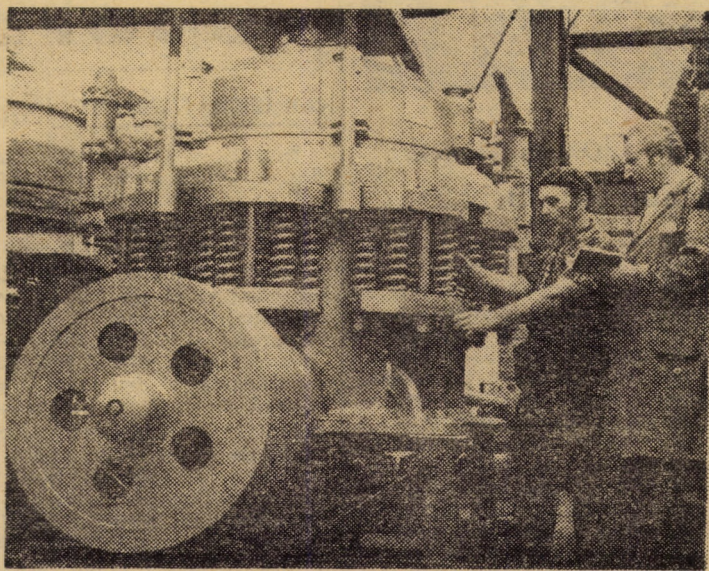
Rampa de expediere a produselor întreprinderii „Independența” Sibiu: maistrul Ilie Dăncăneț și Nicolae Faloba, șef de echipă, efectuind un ultim control la un granulator Ø 900 mm destinat carierelor de piatră
