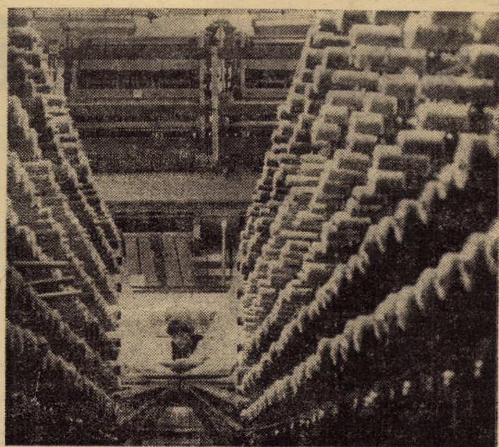
La unul din modernele războaie de țesut, date recent în funcțiune în secția covoare plușate (noua capacitate) la întreprinderea „Textila” Cisnădie
