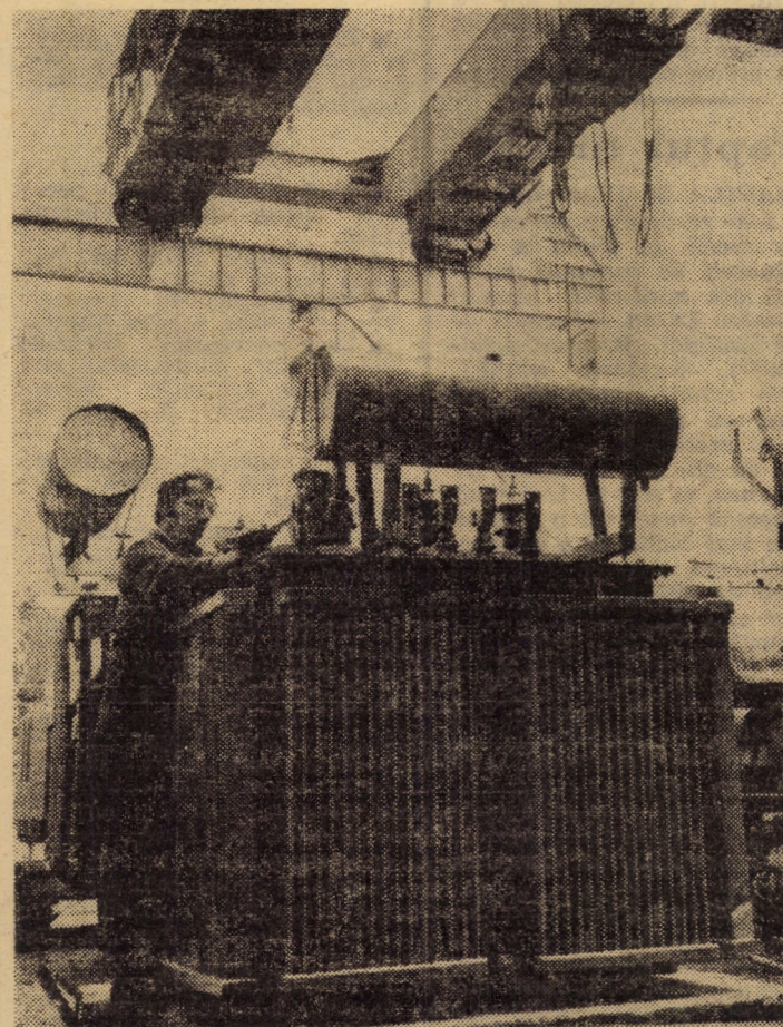
Rampa de încărcare și descărcare a transformatoarelor de mare putere, reparate la I.R.E. Sibiu Foto: FRED NUSS
