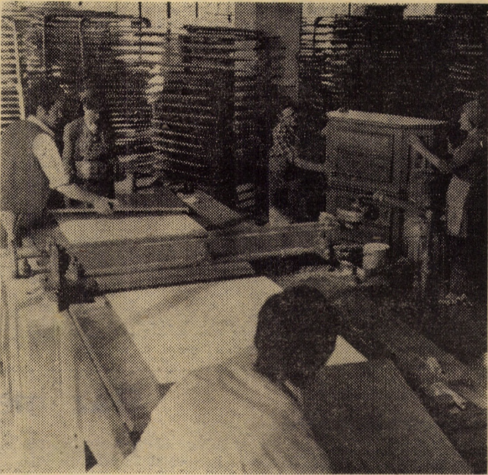
I.P.L. Sibiu — secția II mobilă, sectorul finisaj. Cu ajutorul unei mașini de turnat se asigură o bună uniformitate a peliculei de lac pe întreaga suprafață a componentelor de mobilă
