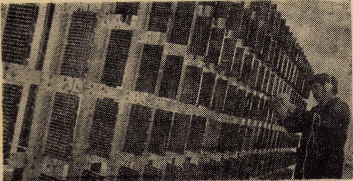
I.R.E. Sibiu. Lucrări de verificare și măsurători profilactice la echipamentele de telemeccanică, aferente dispecerului energetic
