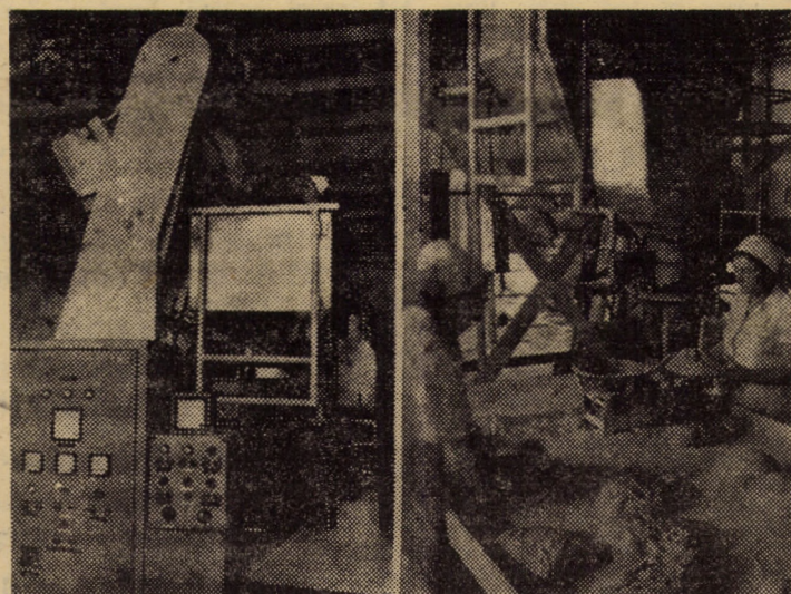
Întreprinderea de morărit, panificație și produse făinoase Sibiu. Prin introducerea unei mașini de divizat aluat pentru piine, realizată prin autodotare, manopera a fost redusă cu 15 la sută
