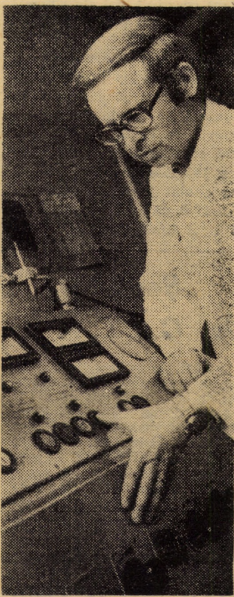
I.C.P.A.O. Mediaș. Aparat de umbră sub vid pentru testarea și prepararea unor probe sub formă de pulbere, deservit de Gheorghe Sălcudean, cercetător științific. Foto: FR. NUSS
