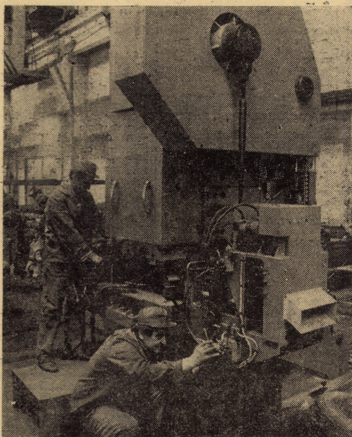
Presa mecanică de 100 tone — se numără printre recente produse realizate de Întreprinderea mecanică Sibiu — utilaj cu un înalt grad de mecanizare a operațiunilor auxiliare.
