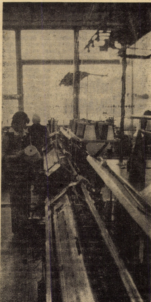
Mașini rectilini automate de tricotat la Fabrica de mănuși și ciorapi Agnita, unitatea Dumbăveni
