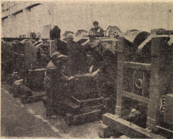
Întreprinderea mecanică Sibiu. Pregătirea unui lot de prese de 63 tone/forță, destinate exportului Foto: FR. NUSS
