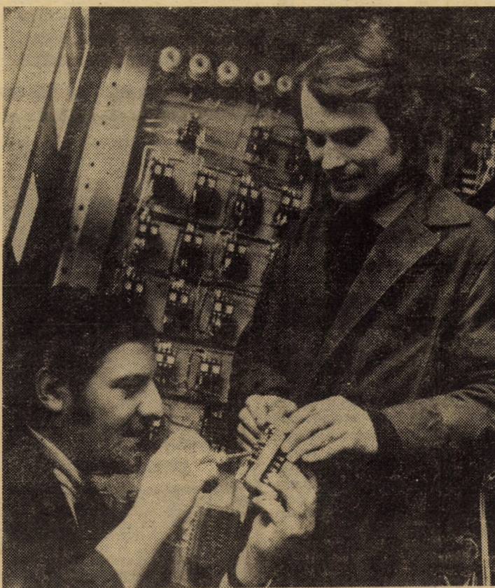
Comuniștii Filon Popa, termotehnician și Dumitru Creștin, electrician, lucrînd la montarea instalațiilor de comandă a noului cuptor de topit cristal cu flux continuu, realizat în cadrul întreprinderii „Vitrometan” Mediaș
