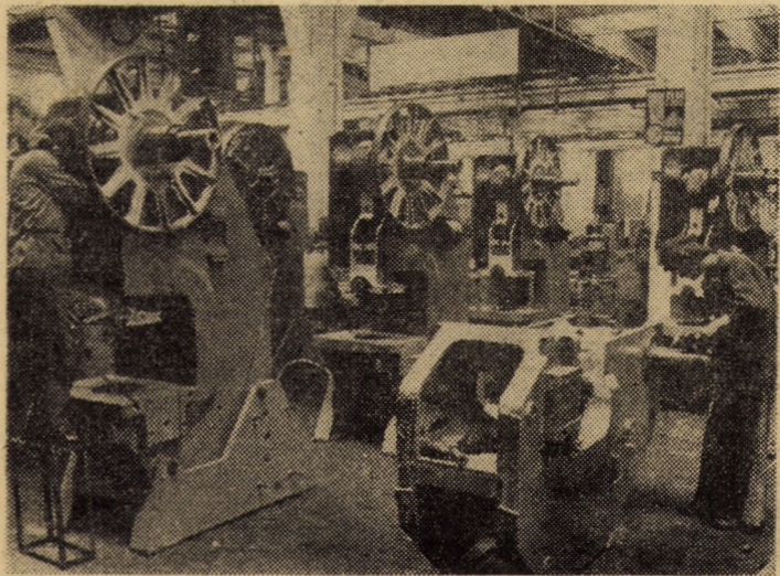
Întreprinderea „Mecanica” Sibiu. Linia de montaj a preselor de 63 tone/forţă — produs destinat exportului
