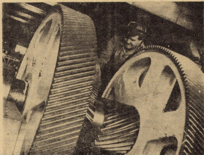
Comunistul Mihai Zalasciuc, șef de echipă în secția utilaj metalurgic a întreprinderii „Independența” din Sibiu, lucrînd la montarea sistemului de angrenaj al reductorului pentru întorcătorul de tablă — produs destinat exportului
