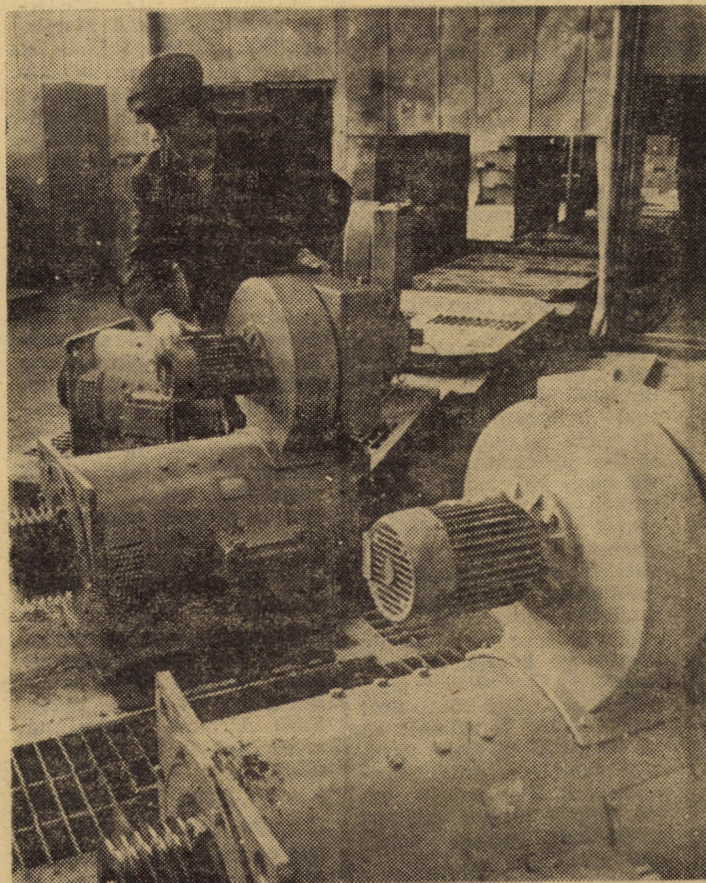
Întreprinderea mecanică Sibiu: mecanisme de acționare pentru mașinile de extrudere politropice, pregătite pentru vopsire Foto: FRED NUSS
