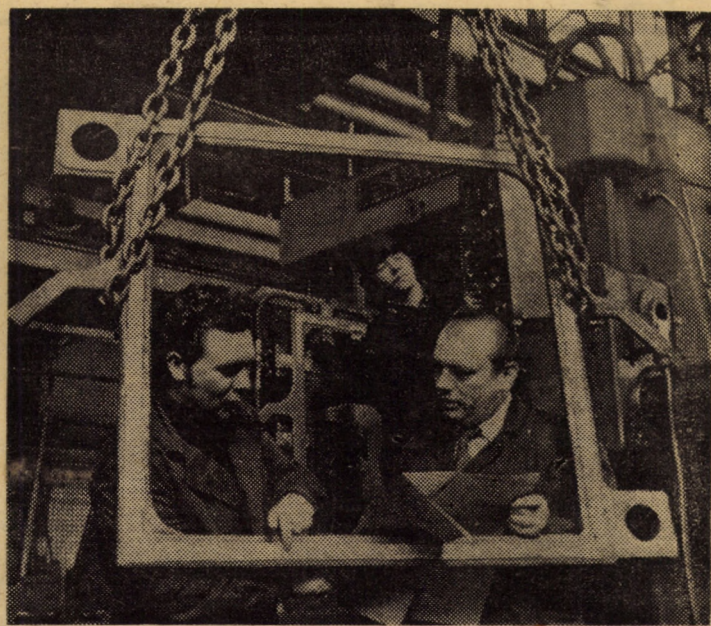
Inginerul Nicolae Boriga și maistrul principal Simion Stoica de la întreprinderea „Independența” Sibiu, analizând calitatea unei rame de la filtru presă, prelucrată după un nou procedeu
