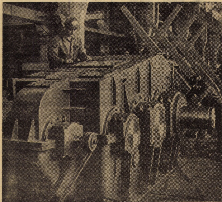
Printre ultimele realizări ale secției utilaj metalurgic de la întreprinderea „Independența” din Sibiu se numără și întorcătorul de tablă. În fotografie reductorul acestui utilaj Foto: FR. NUSS
