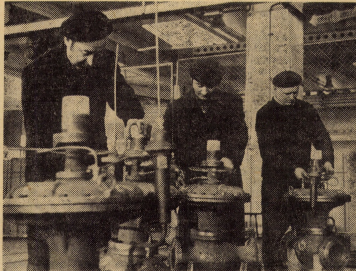
La linia montaj reglatoare de medie presiune — în secția aparate de ardere a Uzinei mecanice gaz metan Mediaș Foto: FR. NUSS
