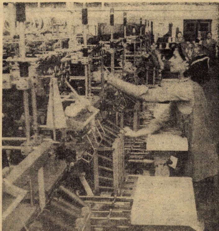
Printre dotările cu utilaje de înaltă productivitate de la „Firul roșu” Tâlmăciu pot fi enumerate și mașinile automate de bătut conice cu patru fuse Foto: FRED NUSS
