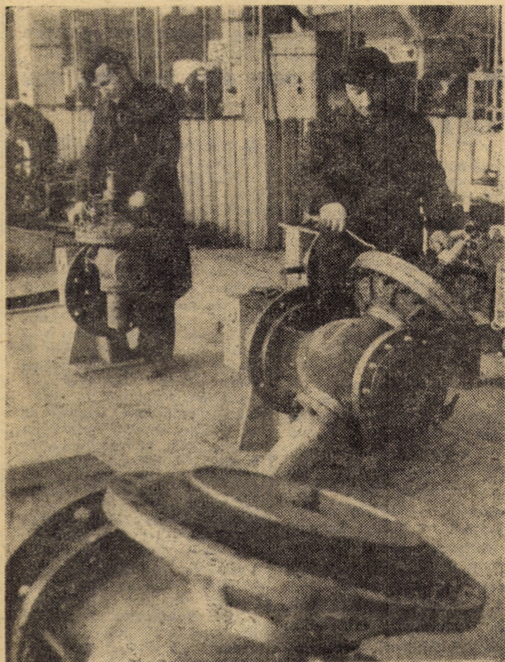
Montajul reguletoarelor de înaltă presiune în secția reguletoare și aparate de ardere de la Uzina mecanică gaz metan Mediaș, efectuat de muncitorii Dumitru Chișu și Emil Mărginean
