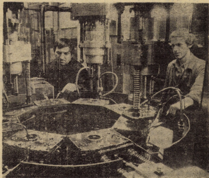
Utilaj realizat prin autoutilare la I.P.A. Sibiu: agregat de prelucrat capace — carcasă a direcției hidraulice. Cu ajutorul lui se execută operații multiple și de înaltă precizie Foto: FR. NUSS
