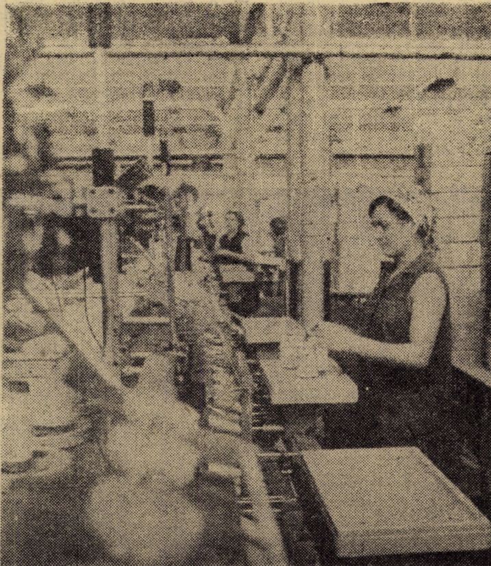
Grupul de mașini de batirat conic — utilaje moderne, de mare randament din secția finisaj a întreprinderii „Firul roșu” Tâlmăciu Foto: FRED NUSS
