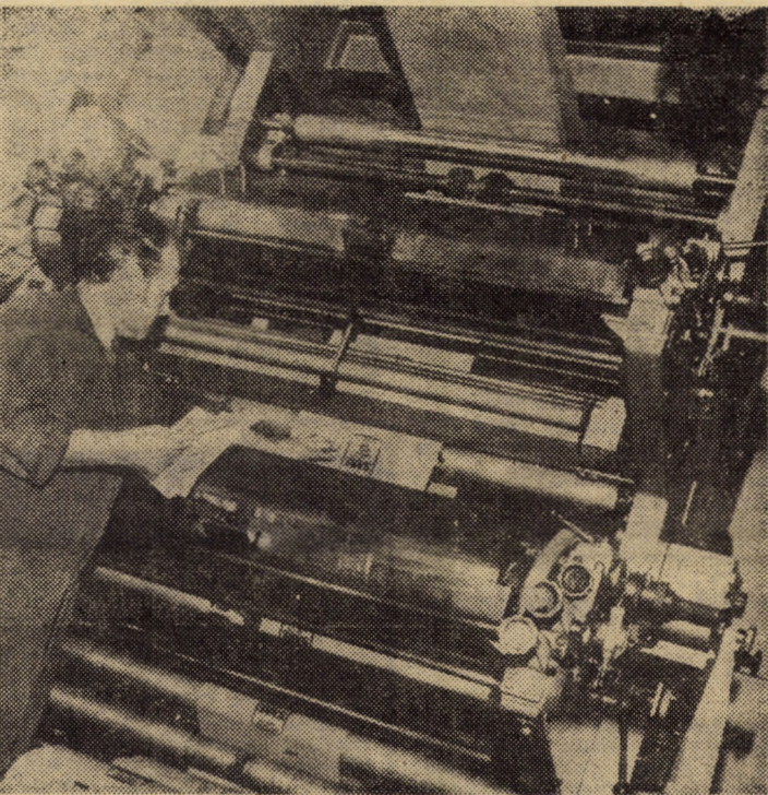
„MIX” Agnita. În cadrul secției mase plastice, o mașină de înalt randament asigură imprimarea în patru culori — după sistem Ofset — a pungilor din polietilenă
