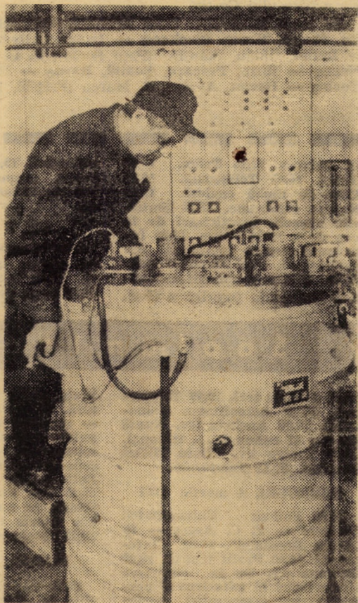
Instalația de ionitrare în cadrul halei de tratare termice de la Întreprinderea mecanică Sibiu Foto: FRED NUSS
