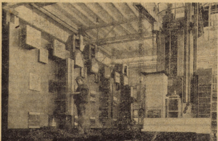
Suportul întorcătorului de tablă — utilaj de mare complexitate, destinat industriei siderurgice, realizat de harnicii constructori ai secției utilaj metalurgic de la întreprinderea „Independența” Sibiu; livrat în prezent și unor beneficiari externi. Foto: H. BÜCHFELNER
