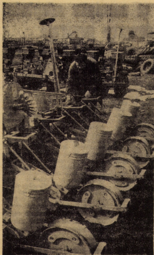
Centrul de reparații al S.M.A. Miercurea Sibului — o ultimă revizie a semănătorilor — reparate și verificate centralizat Foto: FR. NUSS
